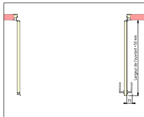
Encombrement vantail 90°
