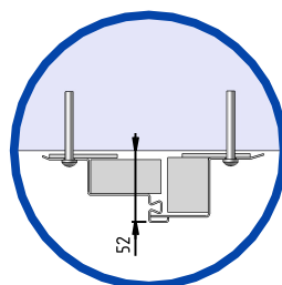
Montage tunnel sur maçonnerie
