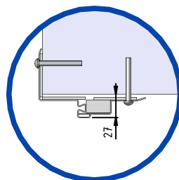
Montage applique sur maçonnerie
