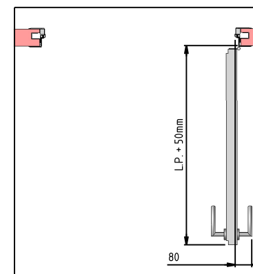
Encombrement vantail 90°
