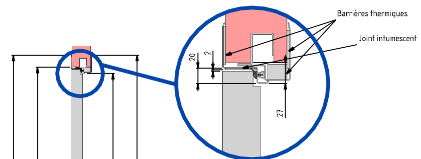
Montage sandwich sur panneaux isothermes LRCF
