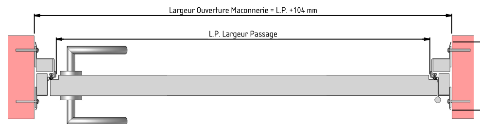
Montage tunnel sur maçonnerie
