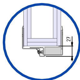
Montage sur placo
