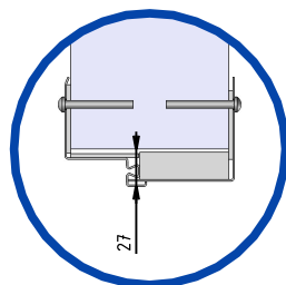
Montage sandwich sur maçonnerie
