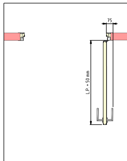
Encombrement vantail 90°
