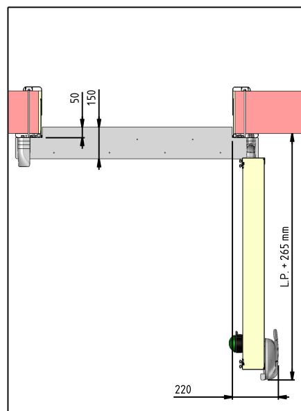
Encombrement vantail 90°
